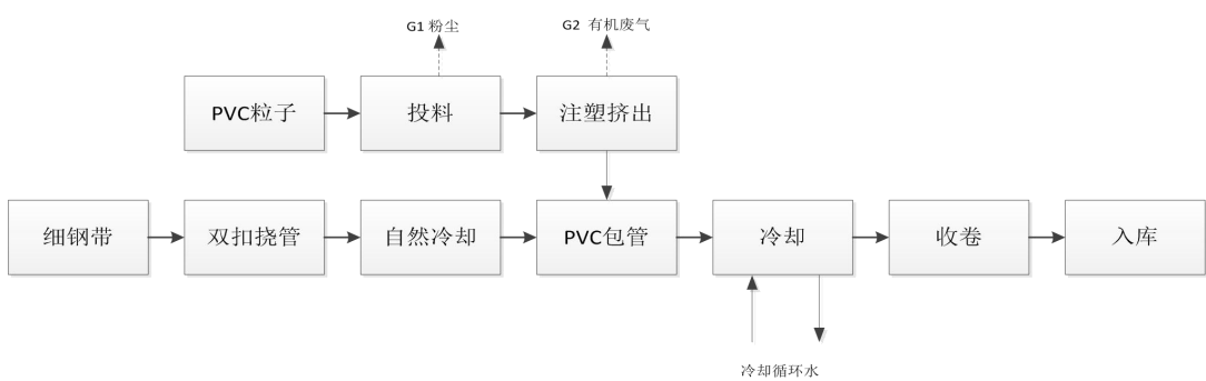
图 1-4 可挠管生产线生产工艺
