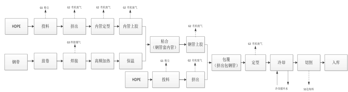
图 1-2 钢塑复合管生产线生产工艺
