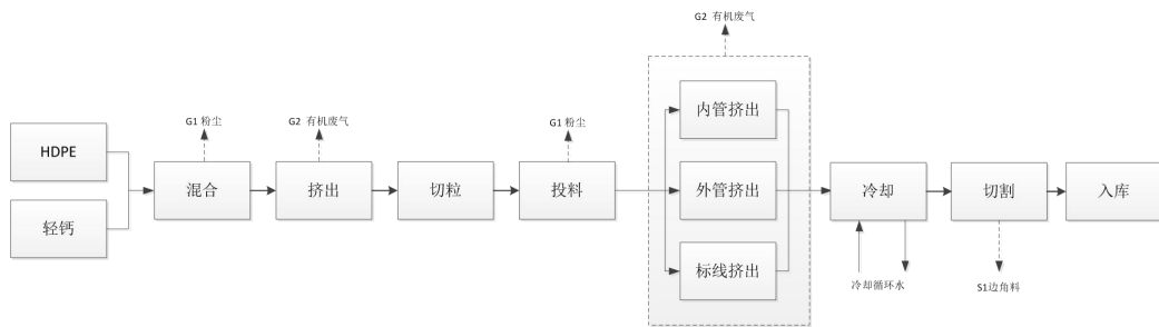
图 1-3 硅芯管生产线生产工艺
